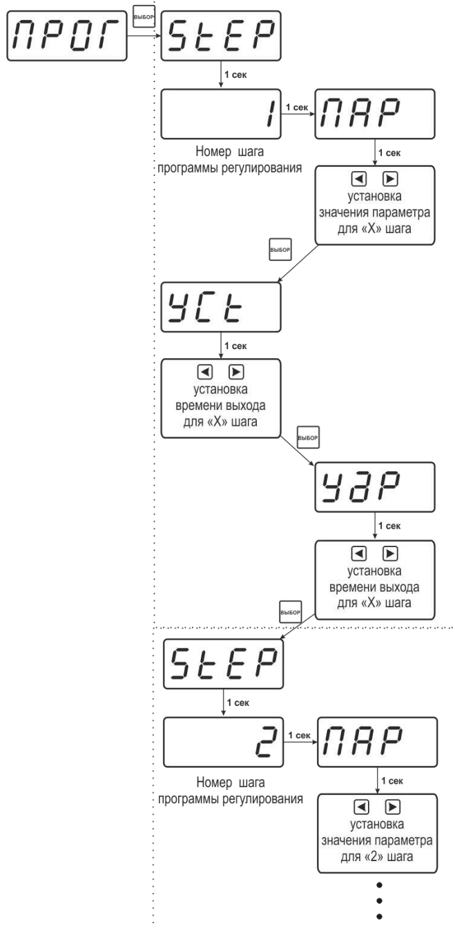
Рисунок 6.20 Программа регулирования
