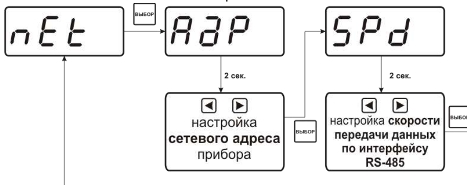
Рисунок 6.22 Меню установки параметров прибора для работы в сети
