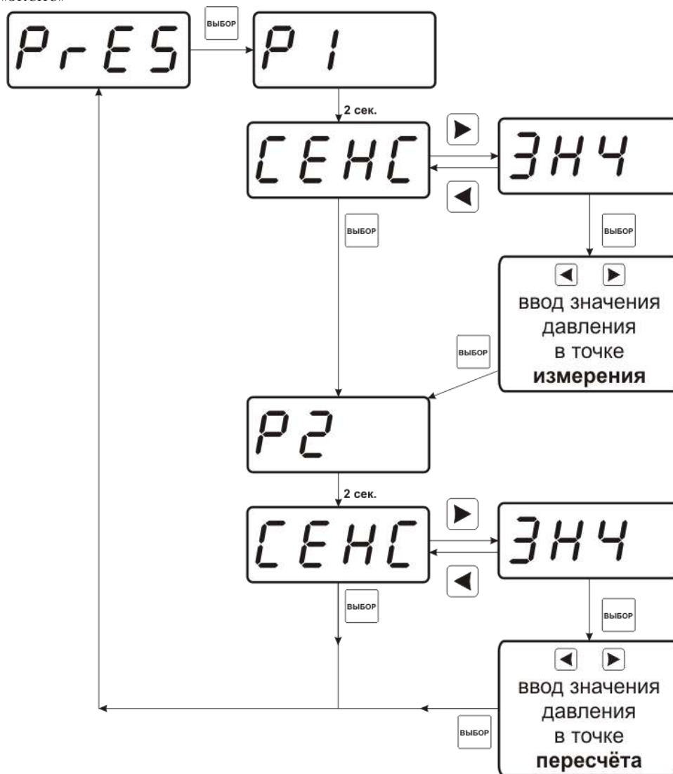
Рисунок 6.9 Схема настройки пересчета влажности
